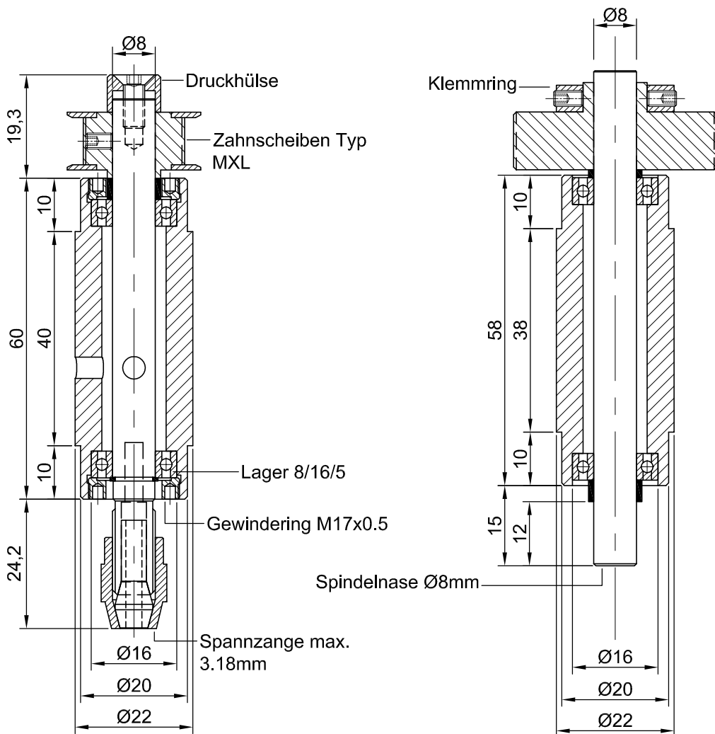
Schnell-Läufer Spindel
